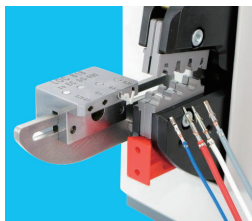
端子定位器 Terminal positioner
