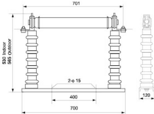
XRNT □ -40.6KV/ □ Fuse base
