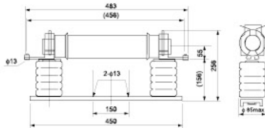
XRNT □ -12KV/ □ Fuse base
