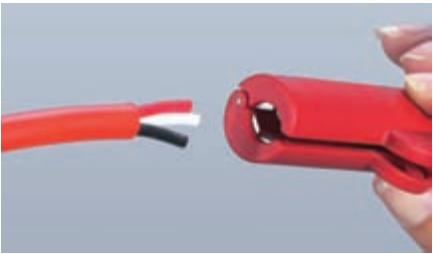
用于 3 \times 0.75\text{mm}^2 的 PVC 圆电缆的剥皮 Stripping used for 3 \times 0.75\text{mm}^2 PVC Circular cable
