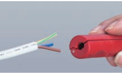
用于 3 \times 0.75\text{mm}^2 的 PVC 圆电缆的剥皮 Stripping used for 3 \times 0.75\text{mm}^2 PVC Circular cable
